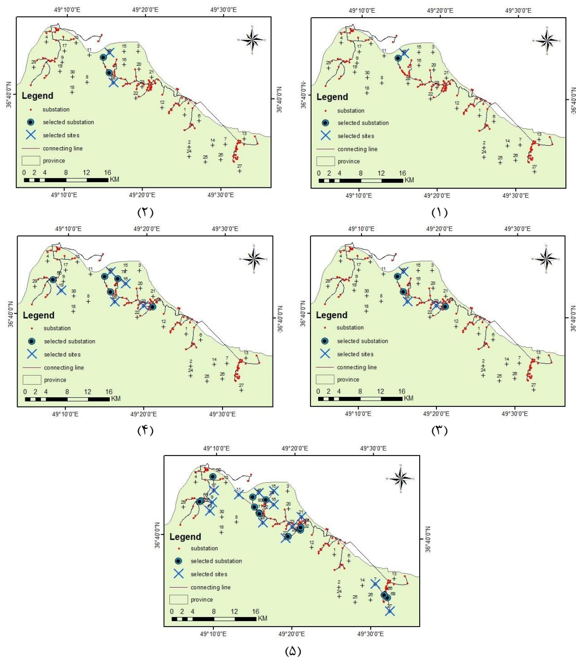
شکل ۸: نمایش مکانی خروجی تخصیص نیروگاه بادی با استفاده از الگوریتم ژنتیک در حالت (۱) نیروگاه بادی، (۲) نیروگاه بادی (۳) نیروگاه بادی (۴) نیروگاه بادی (۵) نیروگاه بادی
