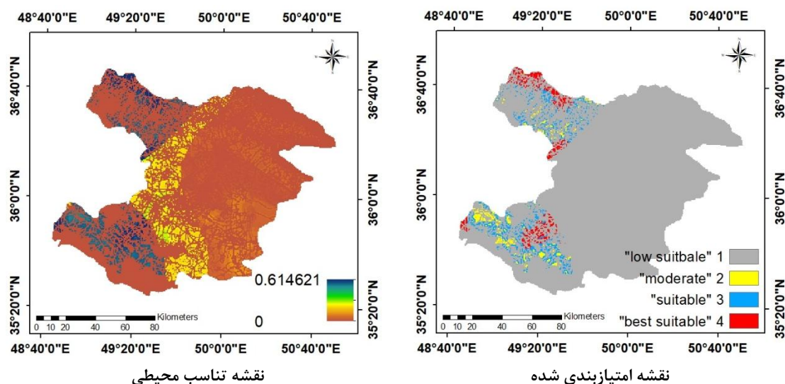
شکل ۴: نقشه‌های نهایی
