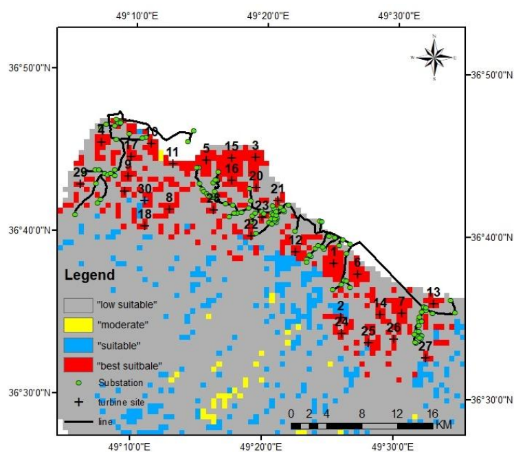
شکل ۵: توزیع مکانی گزینه‌ها و پست‌های برق
