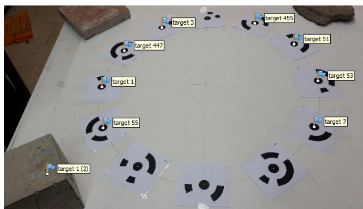
شکل ۱۰: بازشناسی خودکار تارگت‌های کددار تحت عکسبرداری با زاویه ۴۵ درجه در محیط آزمایشگاه
