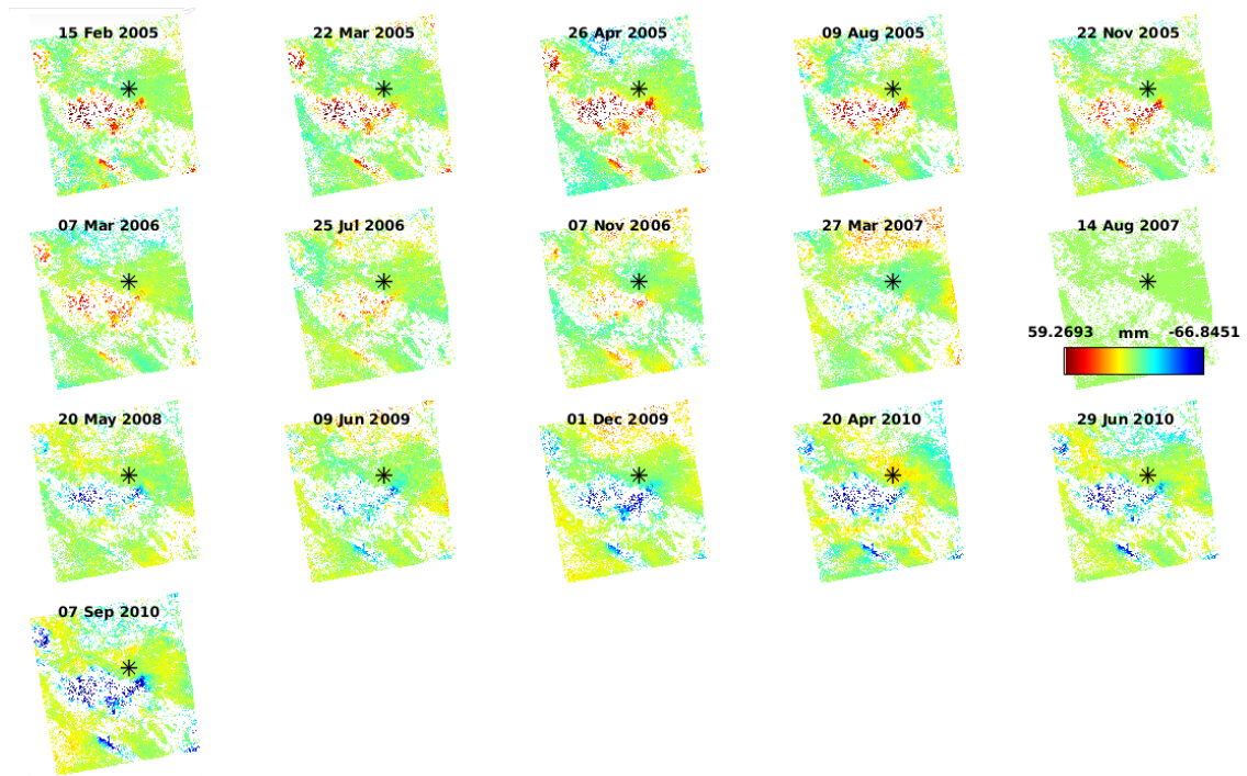
شکل ۶: سری زمانی جابجایی های بدست آمده از InSAR
