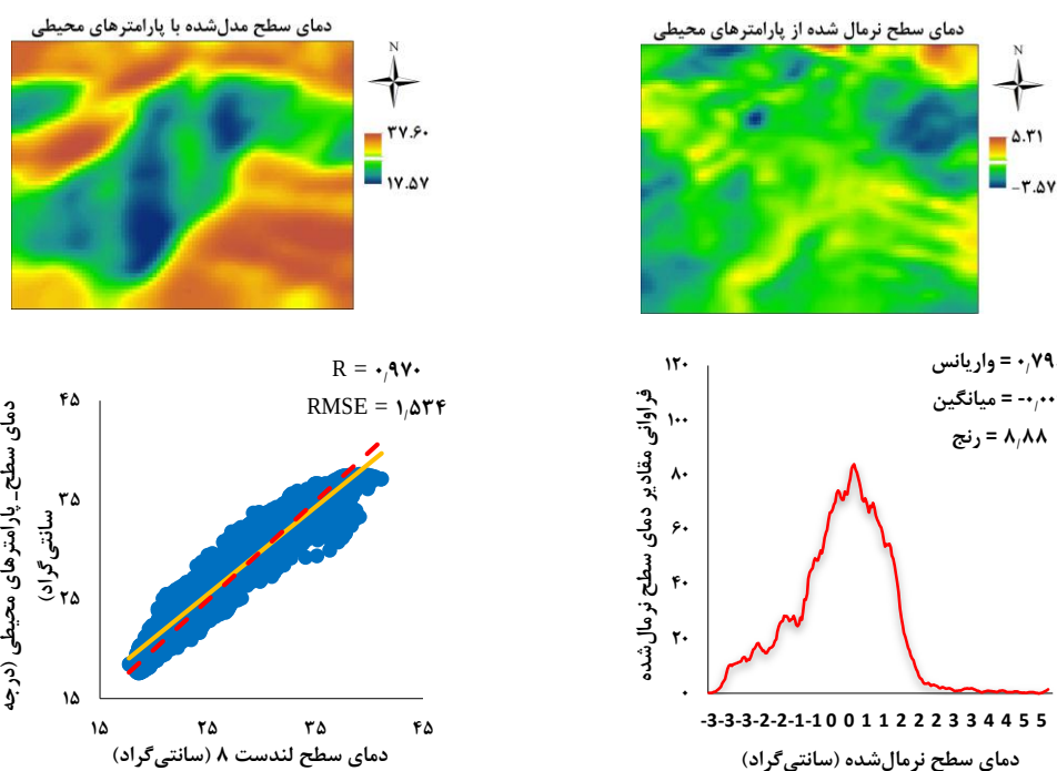
شکل ۱۰: دمای سطح مدل‌شده با توجه به پارامترهای محیطی (سانتی‌گراد)، نمودار فضای ویژگی بین دمای سطح مدل‌شده و دمای سطح مشاهده‌شده، دمای سطح نرمال‌شده از پارامترهای محیطی و هیستوگرام مقادیر دمای سطح نرمال‌شده نهایی
