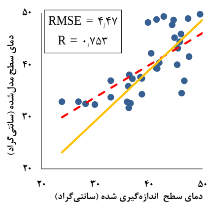
شکل ۱۳: ارزیابی کارایی مدل ارائه شده برای مدل سازی و نرمال سازی دمای سطح با داده‌های زمینی
