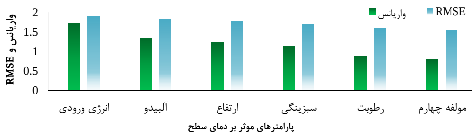
شکل ۹: روند کاهش RMSE و واریانس با اضافه شدن هر پارامتر محیطی به مدل نرمال‌سازی دمای سطح
