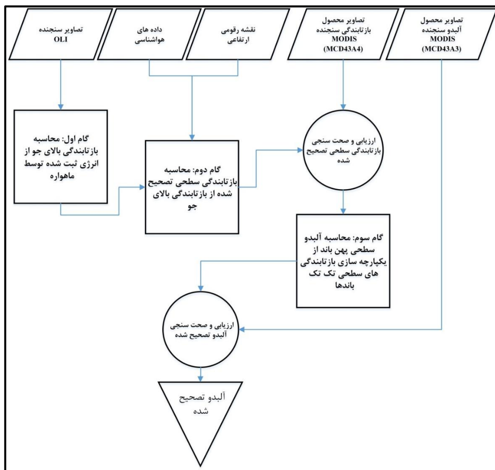
شکل ۲: مراحل برآورد آلبدو تصحیح شده در تحقیق حاضر
