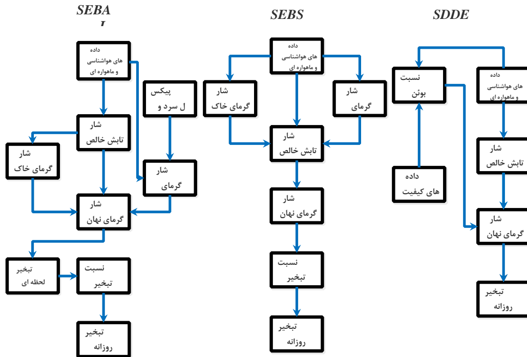
شکل ۲: خلاصه روش محاسباتی برآورد تبخیر با استفاده از سه مدل SEBAL ، SEBS و SDDE
