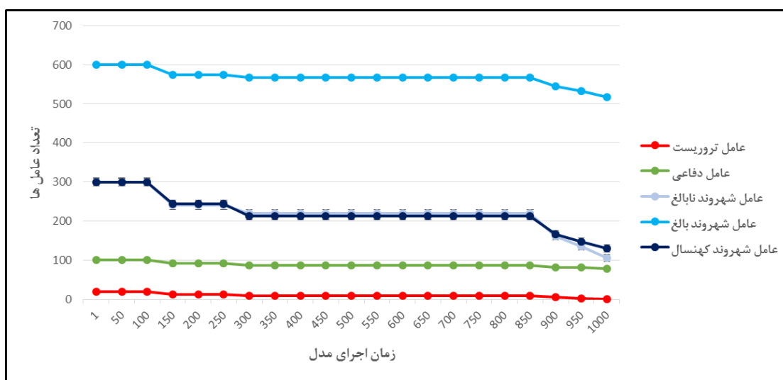
شکل ۷: تعداد عامل‌ها پس از ۱۰۰۰ اجرای مدل عامل‌مبنای تخلیه اضطراری
