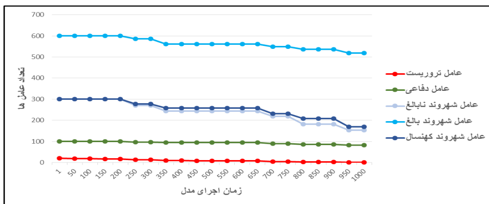
شکل ۱۲: تعداد عامل‌ها در صورت تخصیص ۶۰ درصد تعداد عامل‌های دفاعی به دفاع از نقاط پرجمعیت و ۴۰ درصد آن‌ها به جستجو و کشف عامل‌های تروریست
