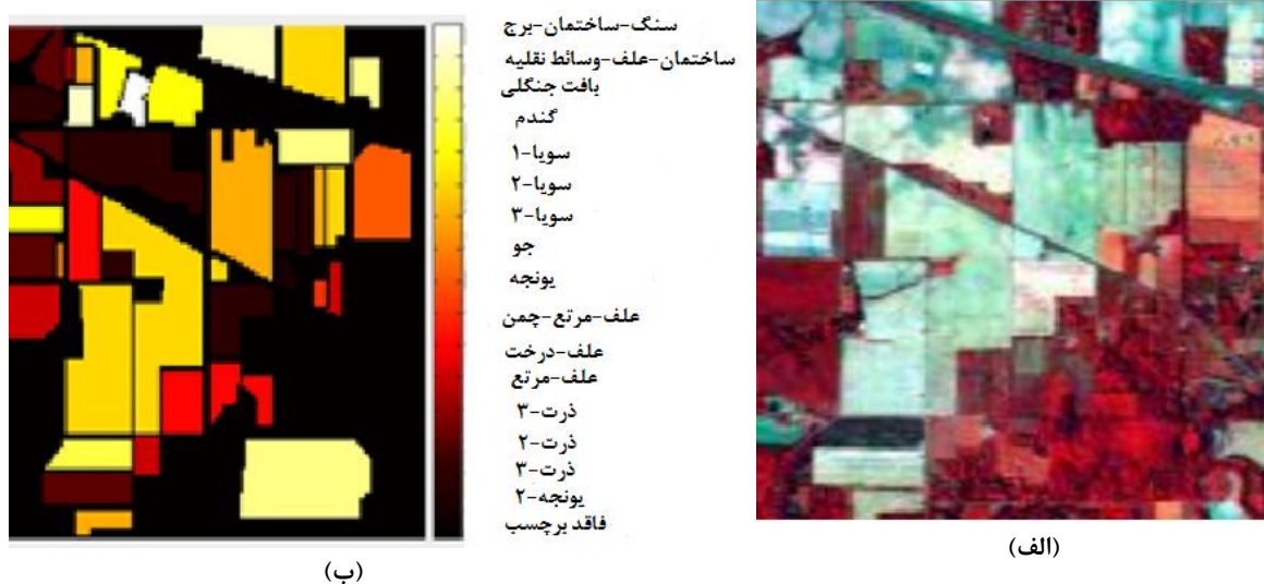
شکل ۴: داده ایندین پائین الف - تصویر رنگی کاذب ب - نقشه واقعیت زمینی
