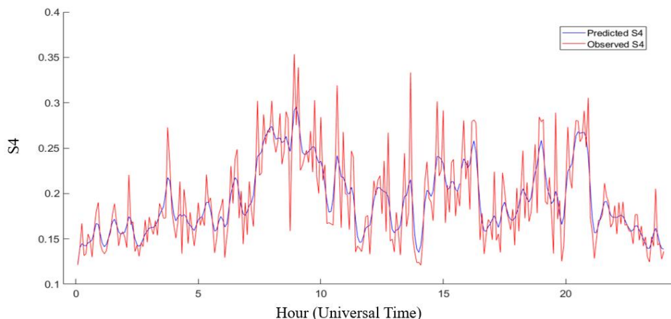
شکل ۱۴: مقایسه میان S_4 پیش‌بینی شده با رنگ آب و S_4 مشاهداتی با رنگ قرمز برای روز اول ماه جولای سال ۲۰۱۷
