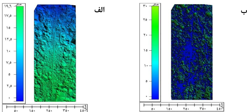
شکل ۴: الف: مدل رقومی سطح زمین ( DTM )، ب: مدل ارتفاعی تاج ( CHM )
