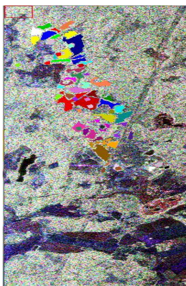
شکل ۳: تصویر پلاریمتری در پایه پاولی، محل مناطق مطلوب بر روی تصویر نشان داده شده است (قرمز= HH-VV ، سبز= HV ، آبی= HH+VV )
