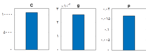
د- نمودار بهینه‌سازی پارامترهای SVR برای تصویر سن‌تینل ۱
