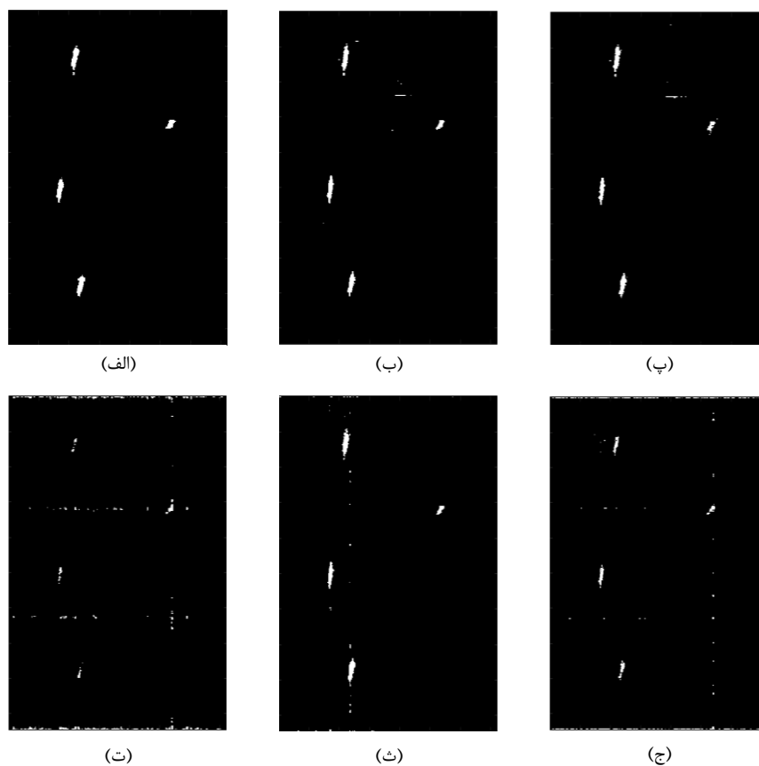
شکل ۸: نتایج آشکارسازی کشتی برای تصویر نشان داده شده در شکل ۵ با استفاده از (الف) روش پیشنهادی \Lambda_N ، (ب) GP ، (پ) PNF ، روش تقارن بازتابی، (ت) 2L-IHP در کانال HH ، (ث) 2L-IHP در کانال HV ، (ج) 2L-IHP در کانال VV .
