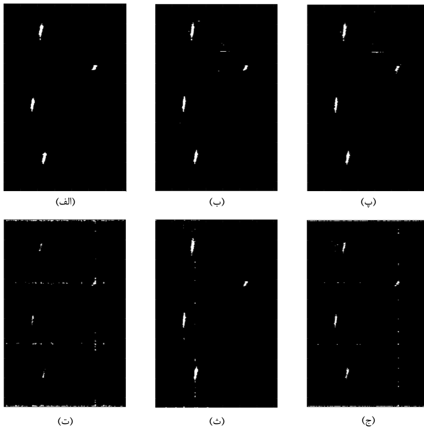
شکل ۸: نتایج آشکارسازی کشتی برای تصویر نشان داده شده در شکل ۵ با استفاده از (الف) روش پیشنهادی \Lambda_N ، (ب) GP ، (پ) روش تقارن بازتابی، (ت) 2L-IHP در کانال HH ، (ث) 2L-IHP در کانال HV ، (ج) 2L-IHP در کانال VV .
