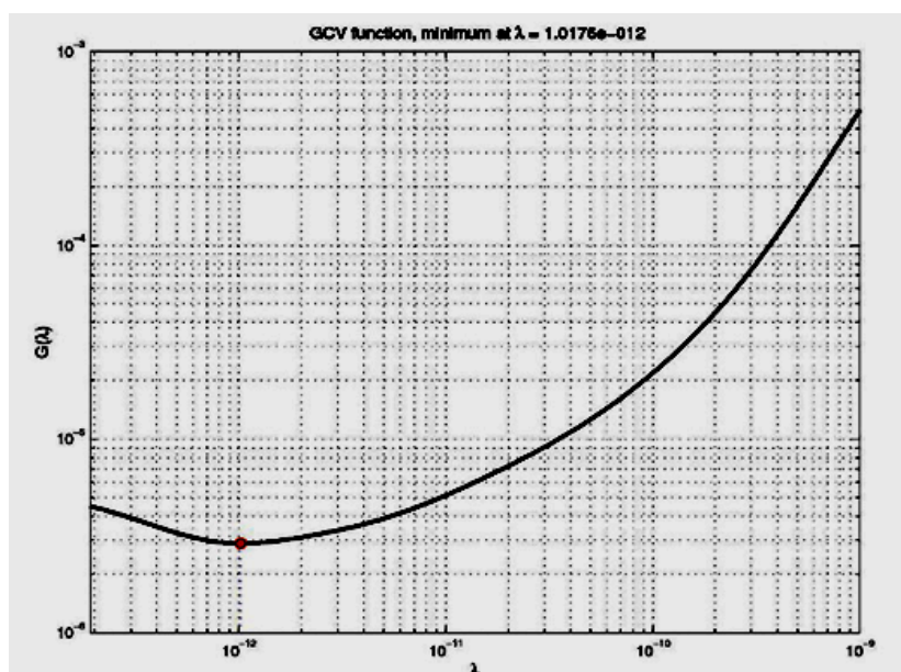
شکل ۸: تابع GCV برحسب پارامتر پایدارساز با مقدار بهینه \lambda = 1.01 \times 10^{-12}
