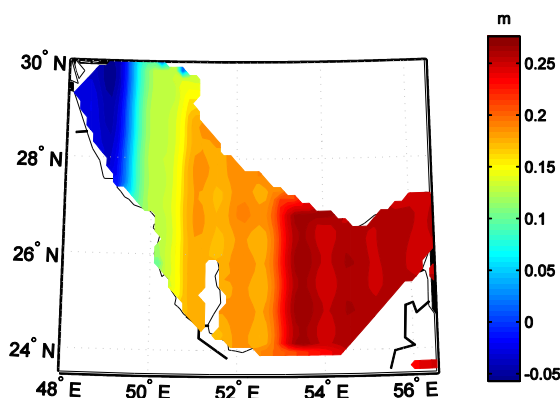
شکل ۲: توپوگرافی سطح دریا در خلیج فارس با استفاده از مدل POCM-4B [22]
