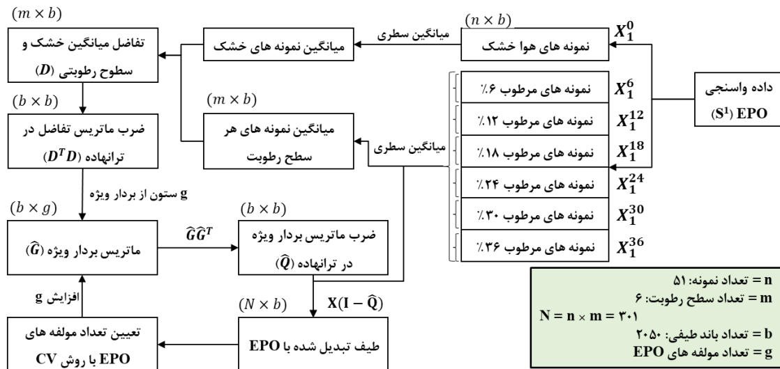
شکل ۳: نحوه پیاده‌سازی الگوریتم EPO برای پارمتر رطوبت.
