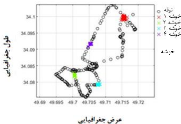
شکل ۵: نقاط توقف استخراج شده توسط روش VDBSCAN با حداقل نقطه برابر ۵۰
