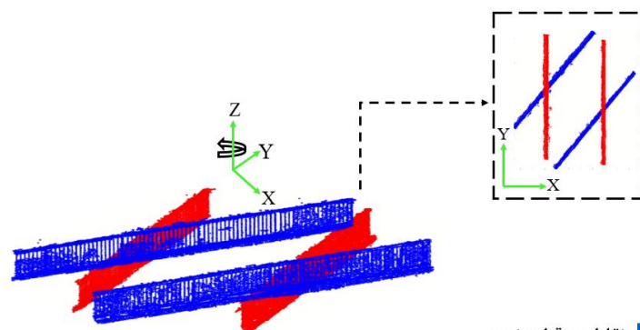
شکل ۳: دوران نقاط هر پل با محاسبه زاویه بین خطوط RANSAC برازش داده شده به نقاط و محور Y
