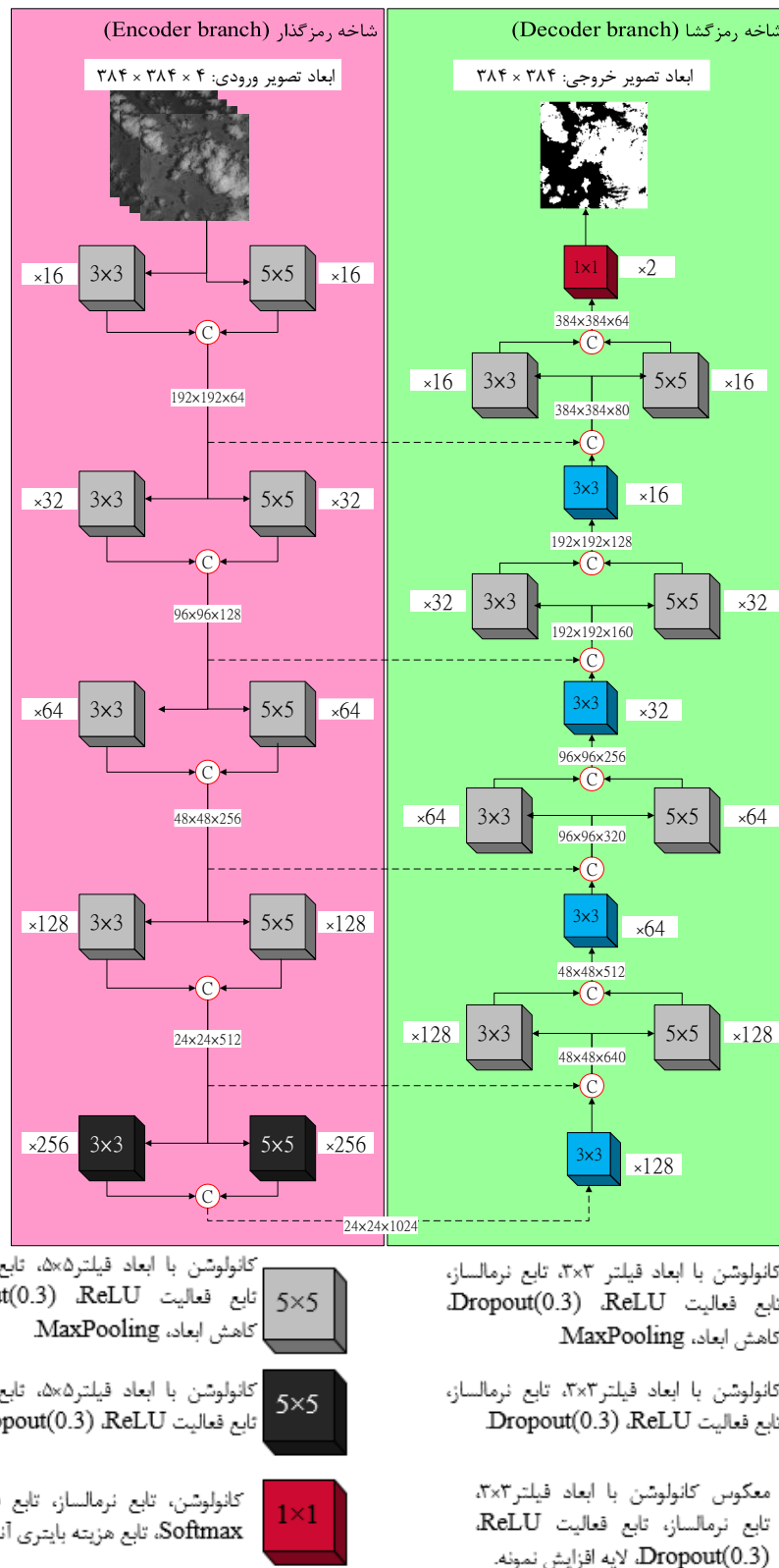
شکل ۲: معماری روش پیشنهادی برای شناسایی ابر در تصاویر ماهواره لندست-۸
