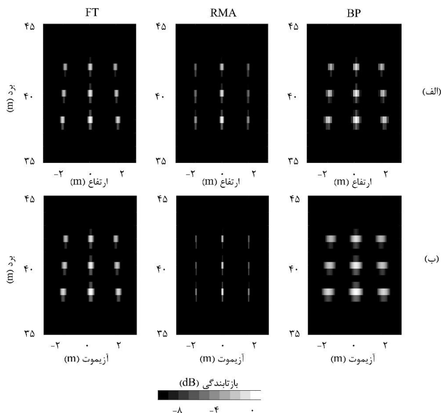
شکل ۵: نتیجه تصویر رادار روزنه مصنوعی اهداف شبیه‌سازی. (الف) در صفحه راستای برد و ارتفاع (صفحه y-z). (ب) در صفحه راستای برد و آزیموت (صفحه y-x)
