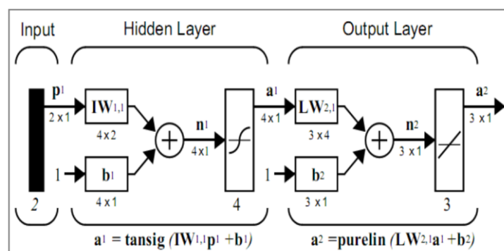
شکل ۱: شبکه عصبی پرسپترون چندلایه
