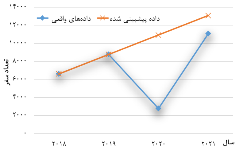
شکل ۱۰: برآورد میزان کاهش تعداد سفر در سال ۲۰۲۰ و ۲۰۲۱
