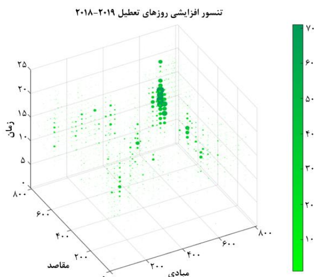
شکل ۱۵: تنسور افزایشی سفرهای تعطیل بین سال ۲۰۱۸ و ۲۰۱۹
