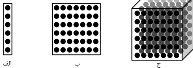
شکل ۲: نمایش ابعاد مختلف جهت ذخیره‌سازی اطلاعات شامل الف: نمایش بردار، ب: نمایش ماتریس و ج: نمایش تنسور سه بُعدی
