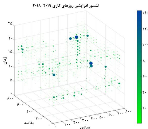
شکل ۱۴: تنسور افزایشی اختلاف سفرهای روزهای کاری بین سال ۲۰۱۸ و ۲۰۱۹
