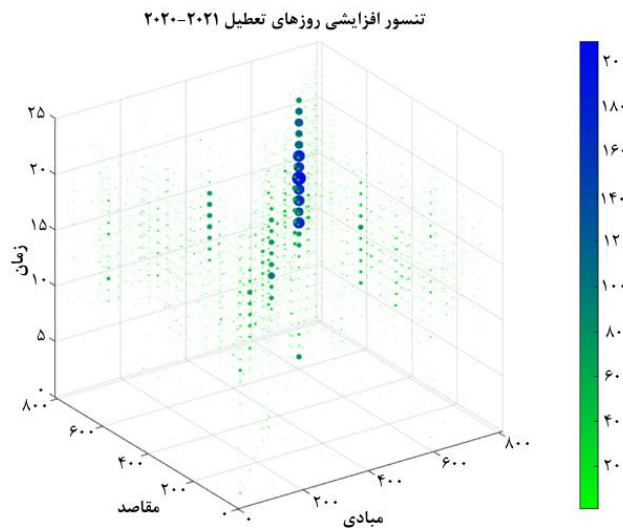
شکل ۱۹: تنسور افزایشی اختلاف سفرهای تعطیل بین سال ۲۰۲۱ و ۲۰۲۰
