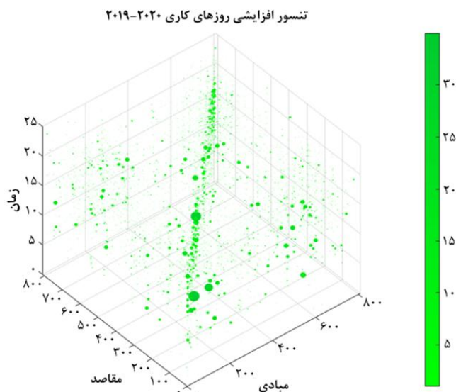
شکل ۱۶: تنسور افزایشی سفرهای روزهای کاری بین سال ۲۰۱۹ و ۲۰۲۰
