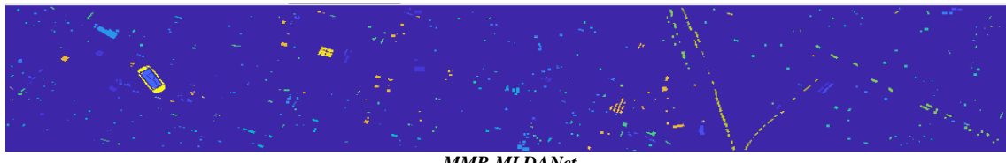
MMP-MLDANet
