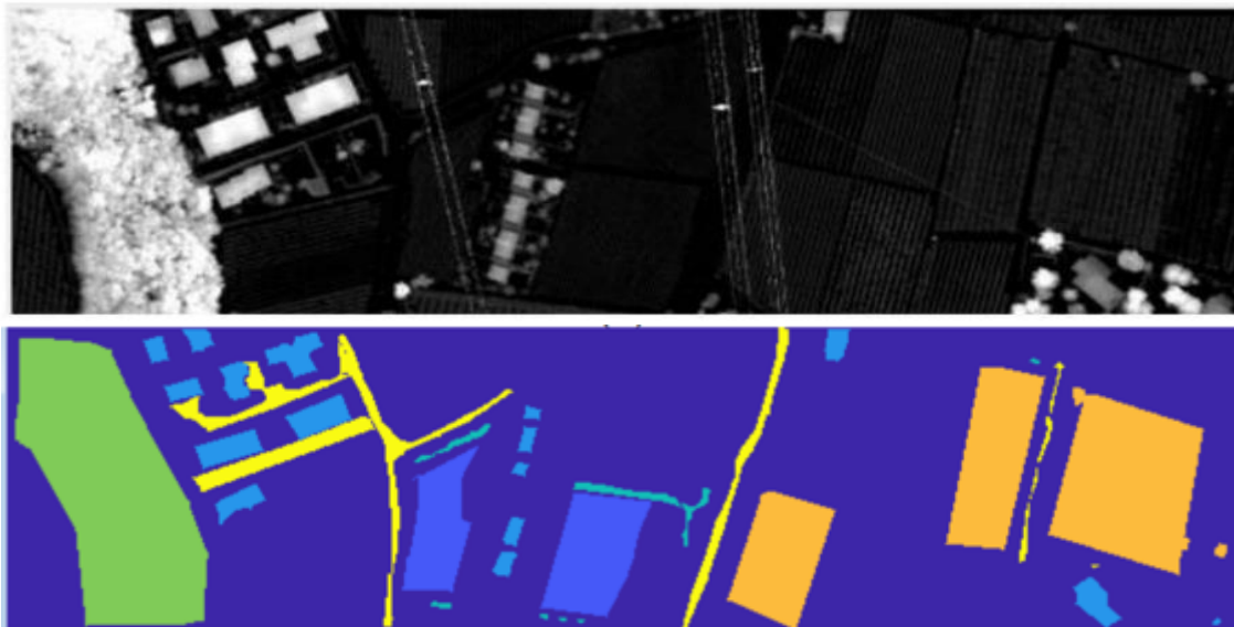
شکل ۴: داده‌ی ترنتو
