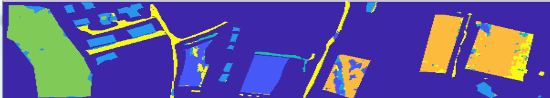
DSM-CNN
