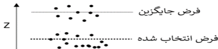
شکل ۶: فرض‌های CUBE
